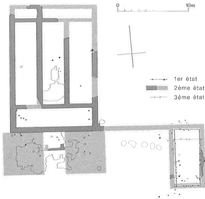
7. Le temple du Kerma Classique (dessins M. Berti, A. Peillex).
